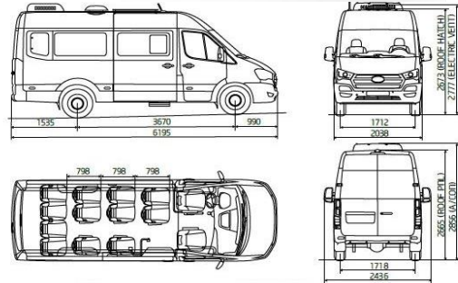
Tolóajtós kivitel
